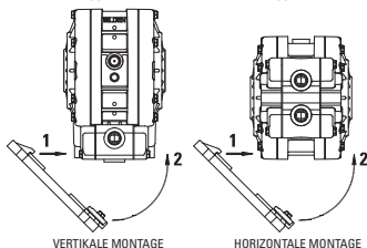
SCHRITT 1 - Befestigungsblock auf Fußbaugruppe (Teil 23) in die gewünschte Nut in der Flüssigkeitskammer (Teil 12) schieben.
