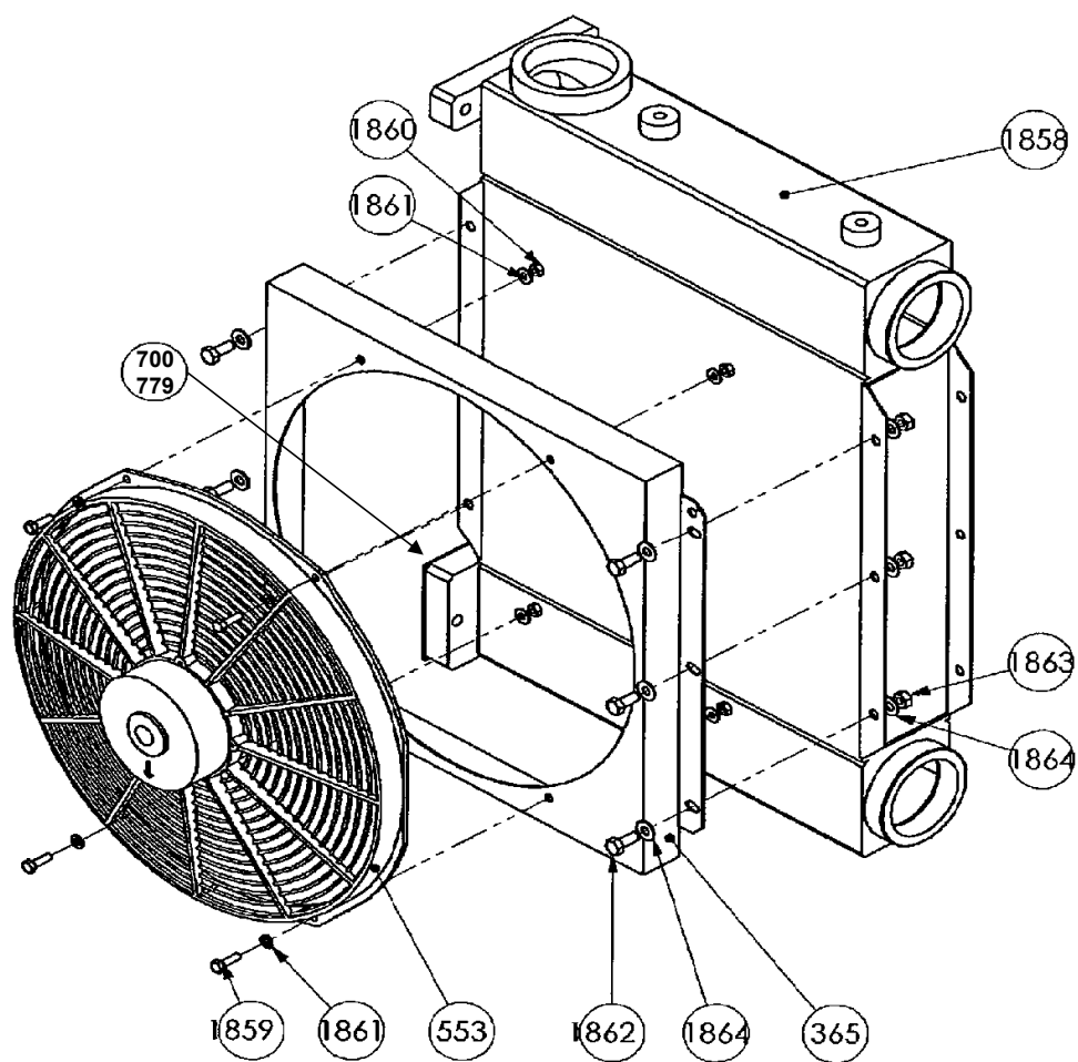
Echangeur
