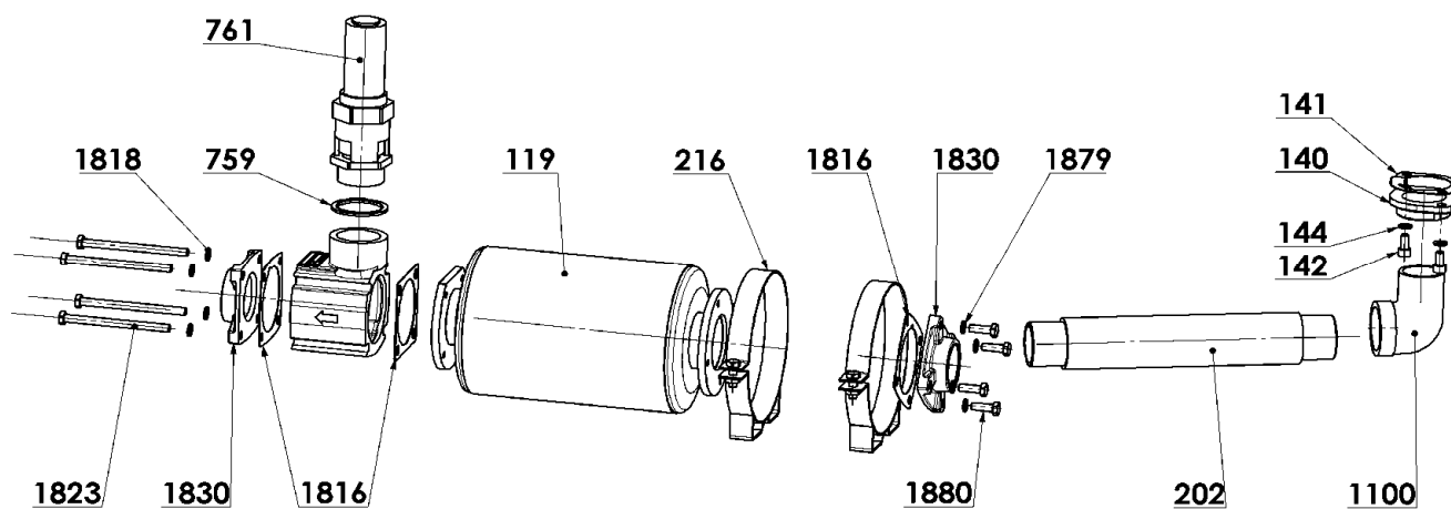
Silencieux
