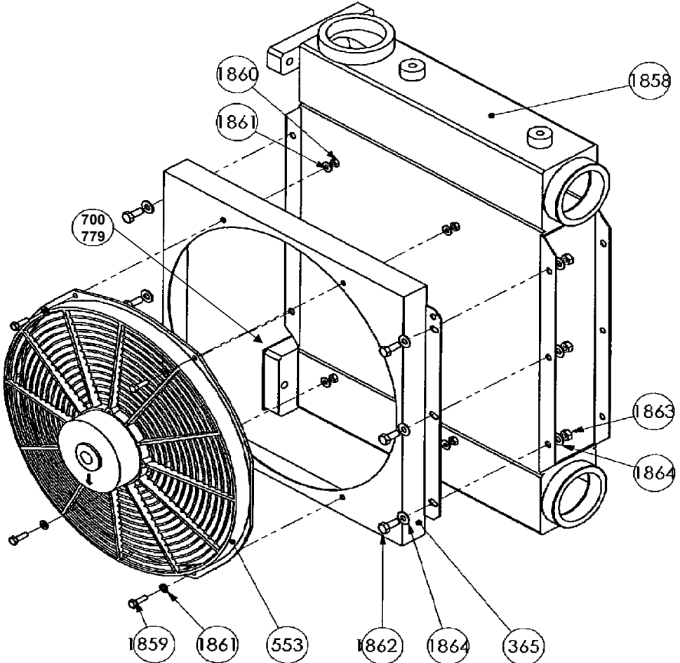
Lüftkuhler
