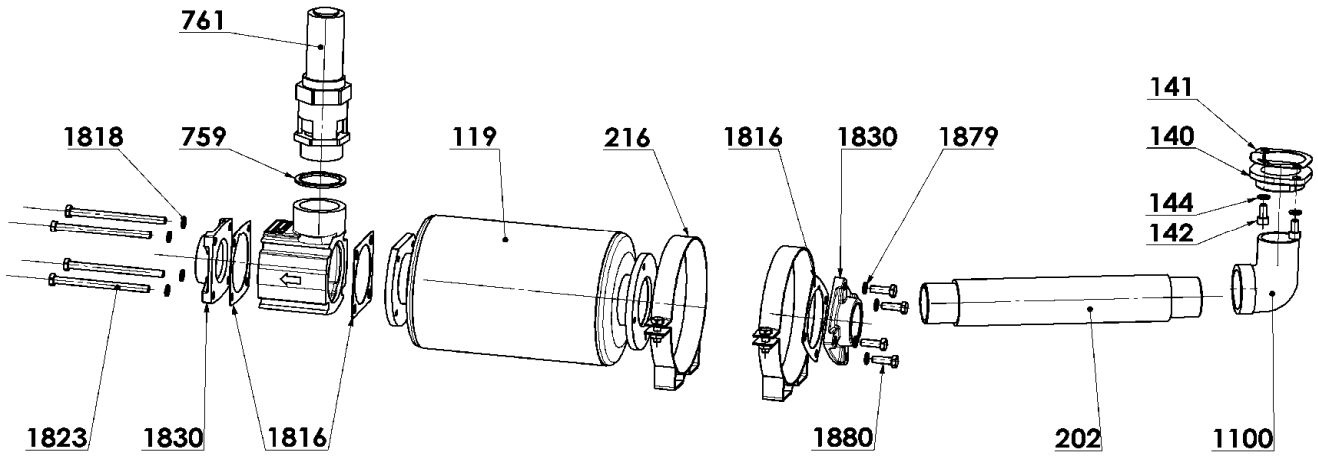
Schalldämpfer
