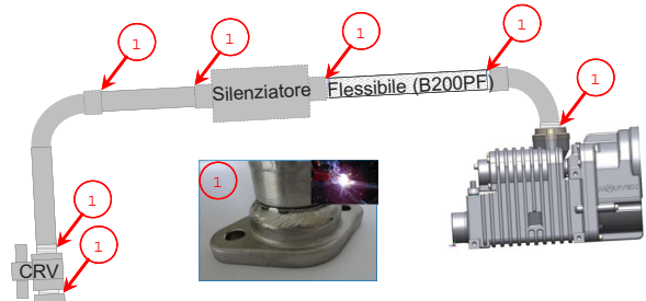
Regole di installazione: Linea di scarico
