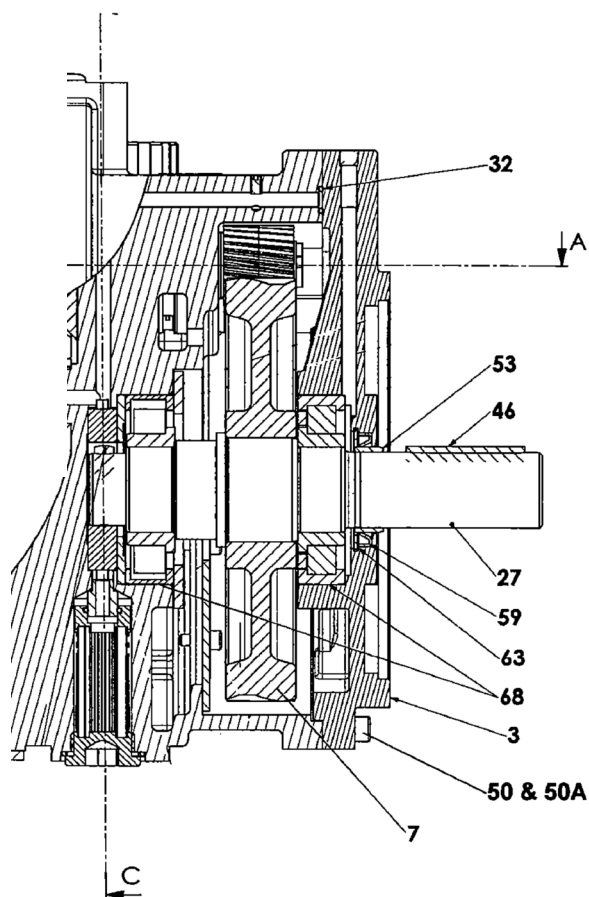
Vue de l'avant du compresseur
