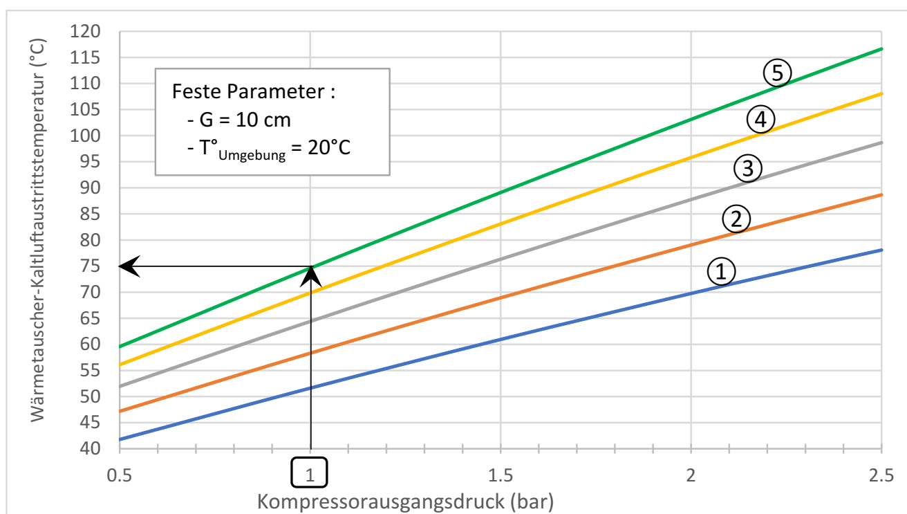
Diagramm A : Einfluss des Kompressoraustragsdrucks auf die Wärmetauscher- Austrittstemperatur
