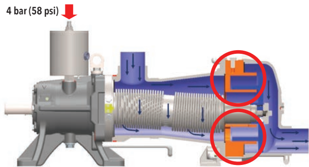
Durch Druckluft im Antriebsblock wird der Faltenbalg gestreckt; der Kolben wird aus dem Zylinder gedrückt.
