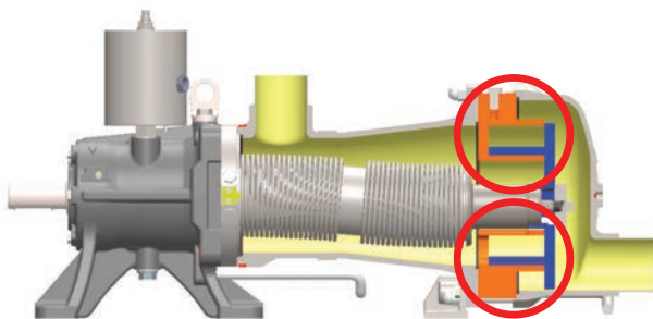
Bei atmosphärischem Druck im Antriebsblock ist der Kolben in Kontakt mit dem Zylinder
