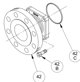
ANSI 3" 300 lb. R.F.
