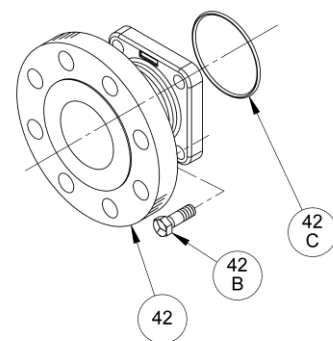
ANSI 2" 300 lb. R.F.
