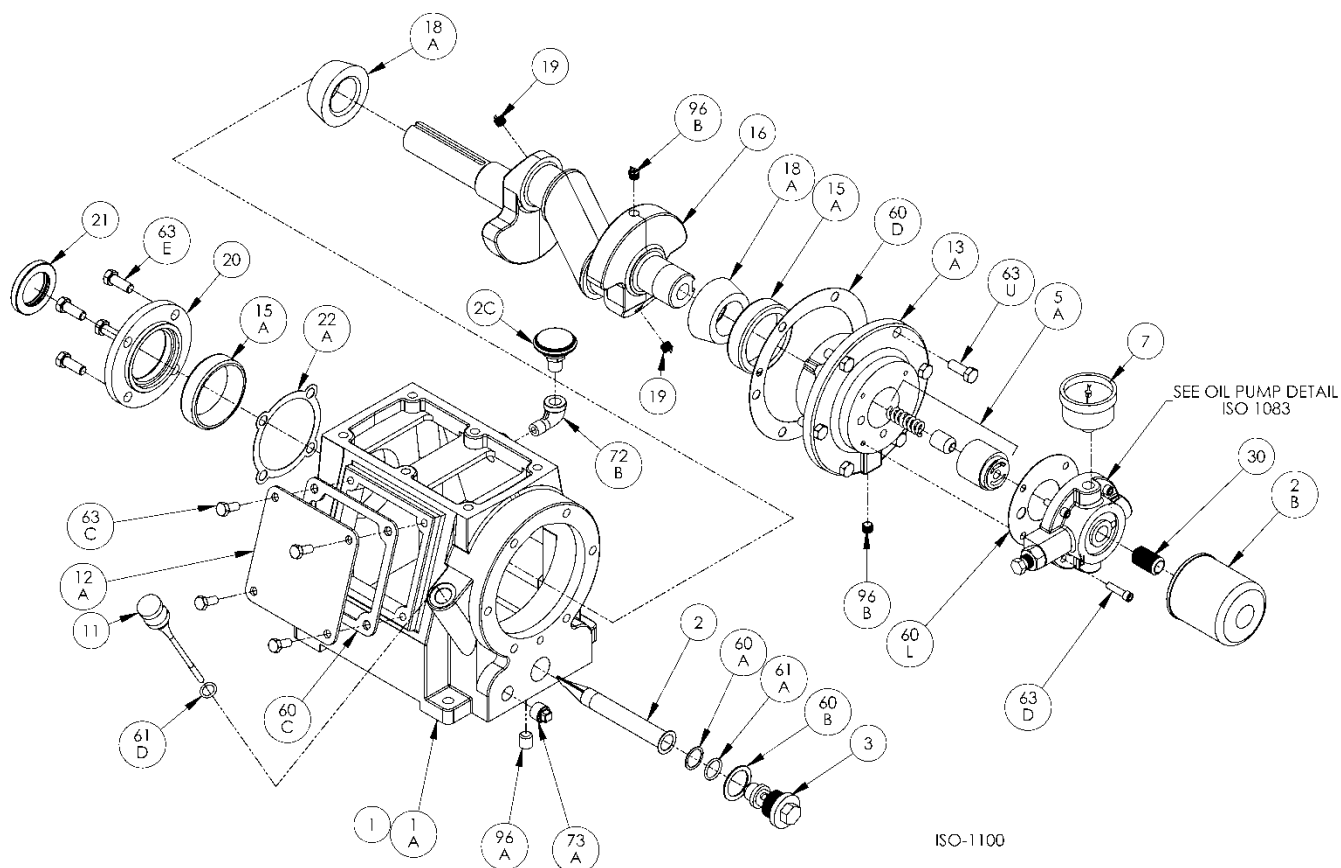
Crankcase: ISO1100
