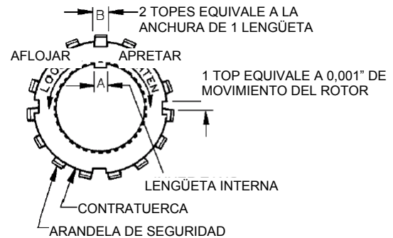
Figura 7 Ajuste de la contratuerca
