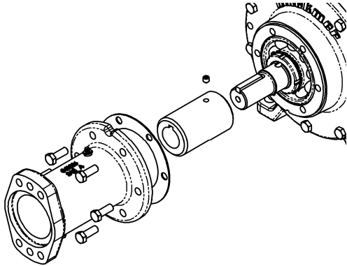
Figura 3 Accionamiento hidráulico
