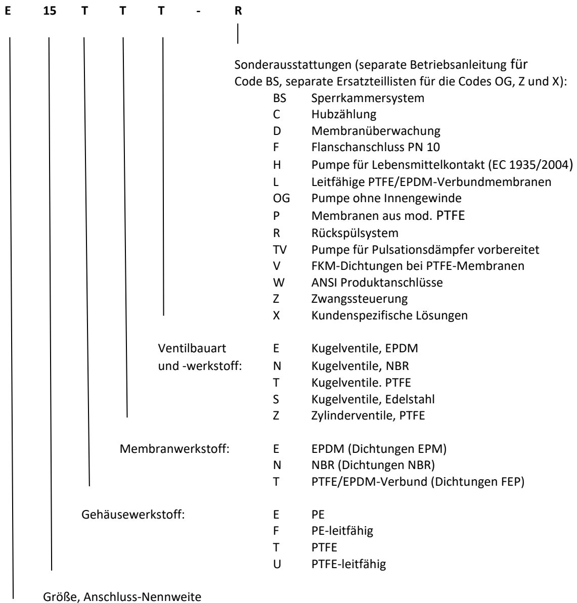
ALMATEC Druckluft-Membranpumpe, E-Serie
