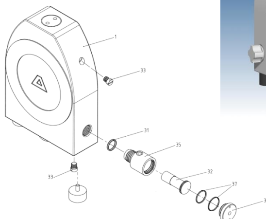
pneumatisches Rückpülsystem (Code R 3 / R 4 / R 6)
