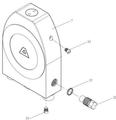
manuelles Rückpülsystem (Code R 1 / R 2 / R 5)
